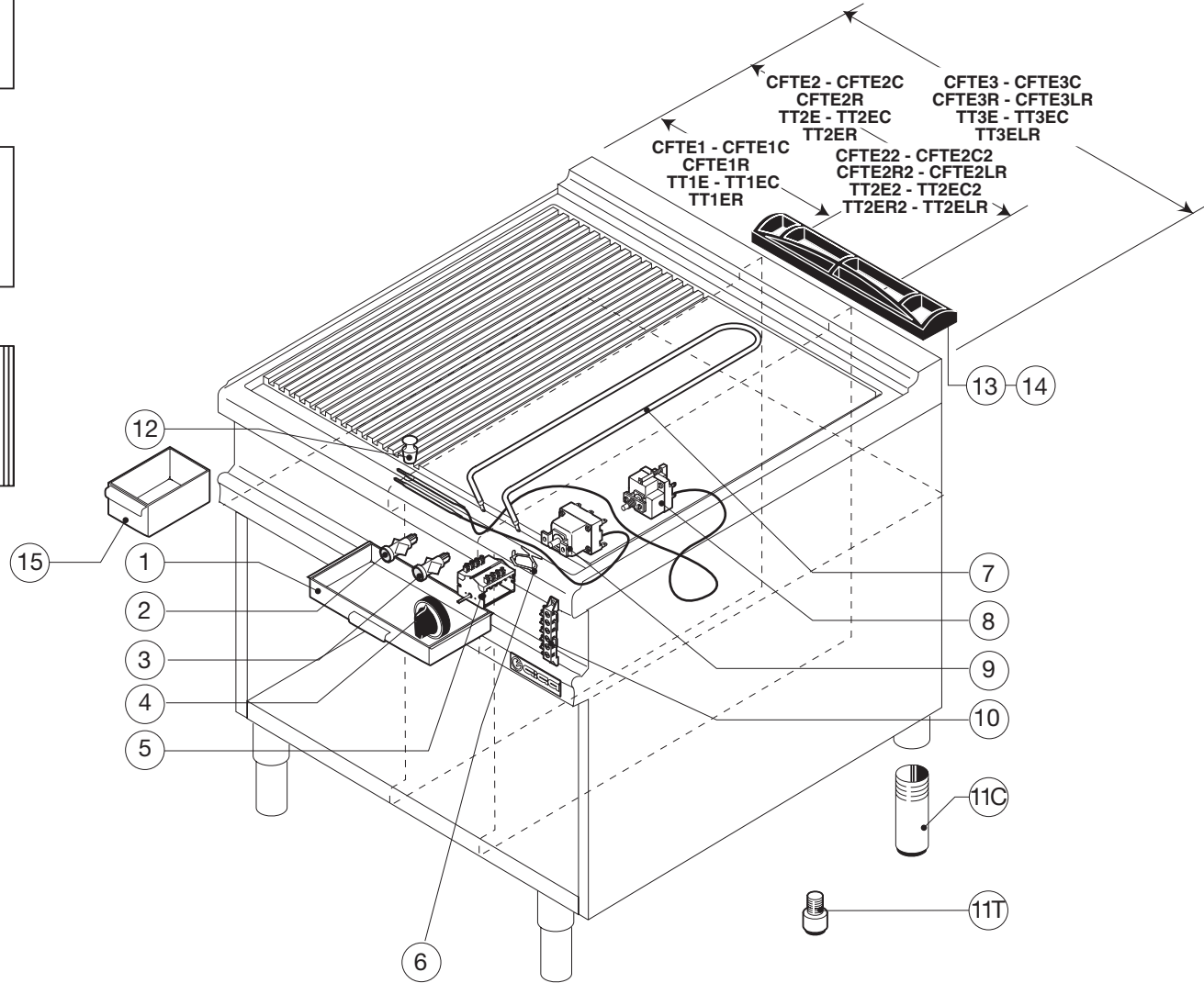
CFTE1 TT1E CFTE2 - TT2E CFTE22 - TT2E2 CFTE3 TT3E
