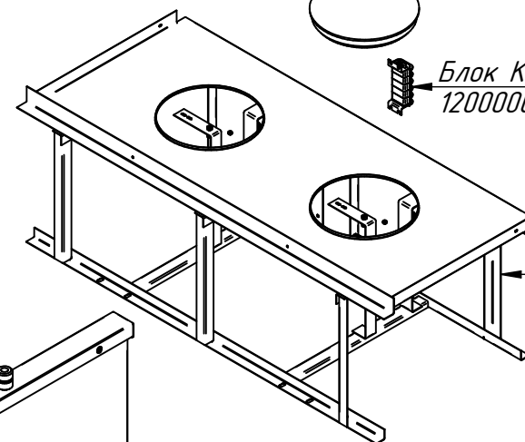
Каркас (в сборе) ПМЭС70Т.1028.04.00.000СБ 21000802646
