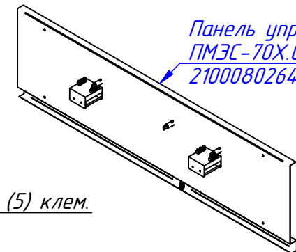
Каркас (в сборе) ПМЭС70Т.1028.04.00.000СБ 21000802646
