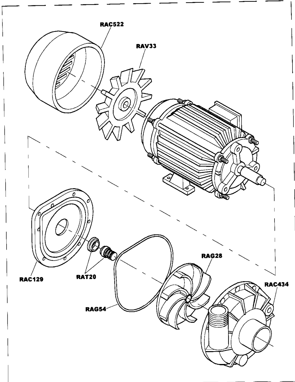
DPE453D DPE453S
