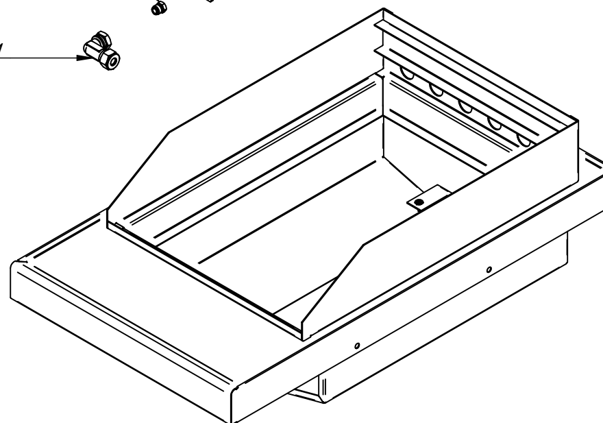
Пилотная форсунка D 0,35 мм (природный газ) 12000046079 Пилотная форсунка D 0,25 мм (сжиженный газ) 12000069410
