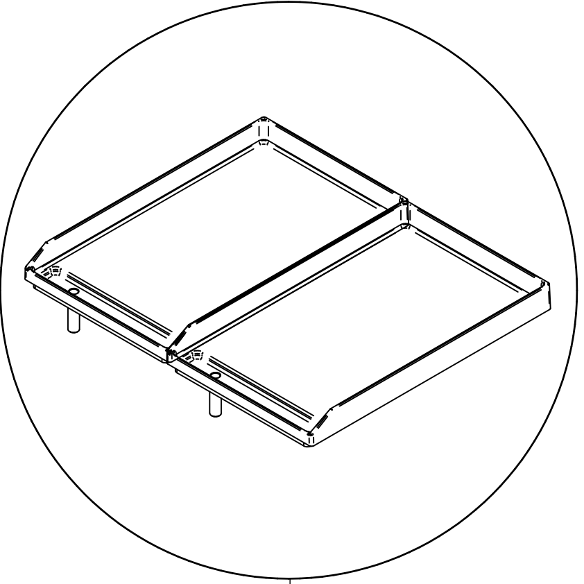
Для ГАЗО-80/2Н-4-01 ГАЗО-80/2Н.1587.00.00.000-01 СБ
