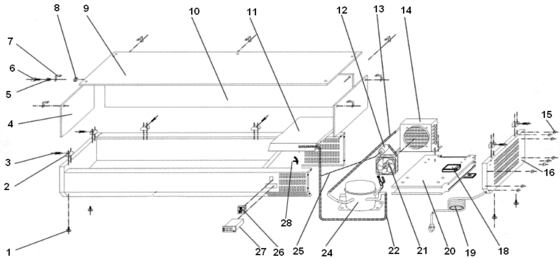
EXPLODE OF RI 330/120-140-150-180-200 RI 380/120-140-150-180-200
