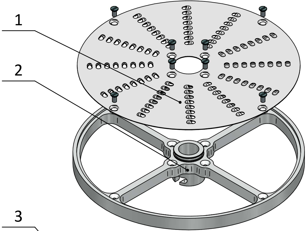
Нож шинковочный 2 мм 410000011489
